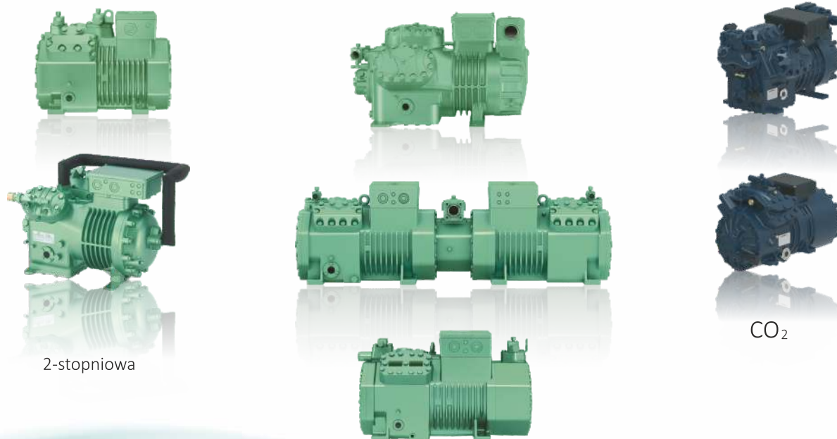
CO 2
