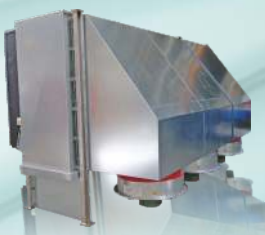
PLKs
