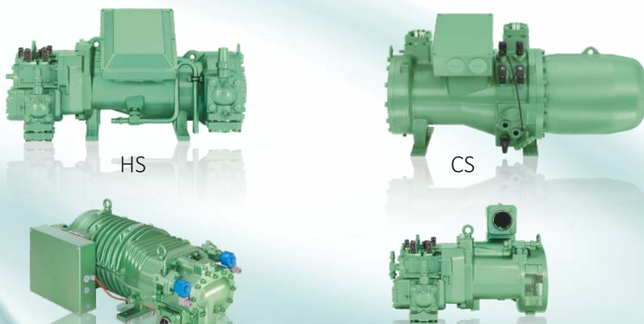
OS
